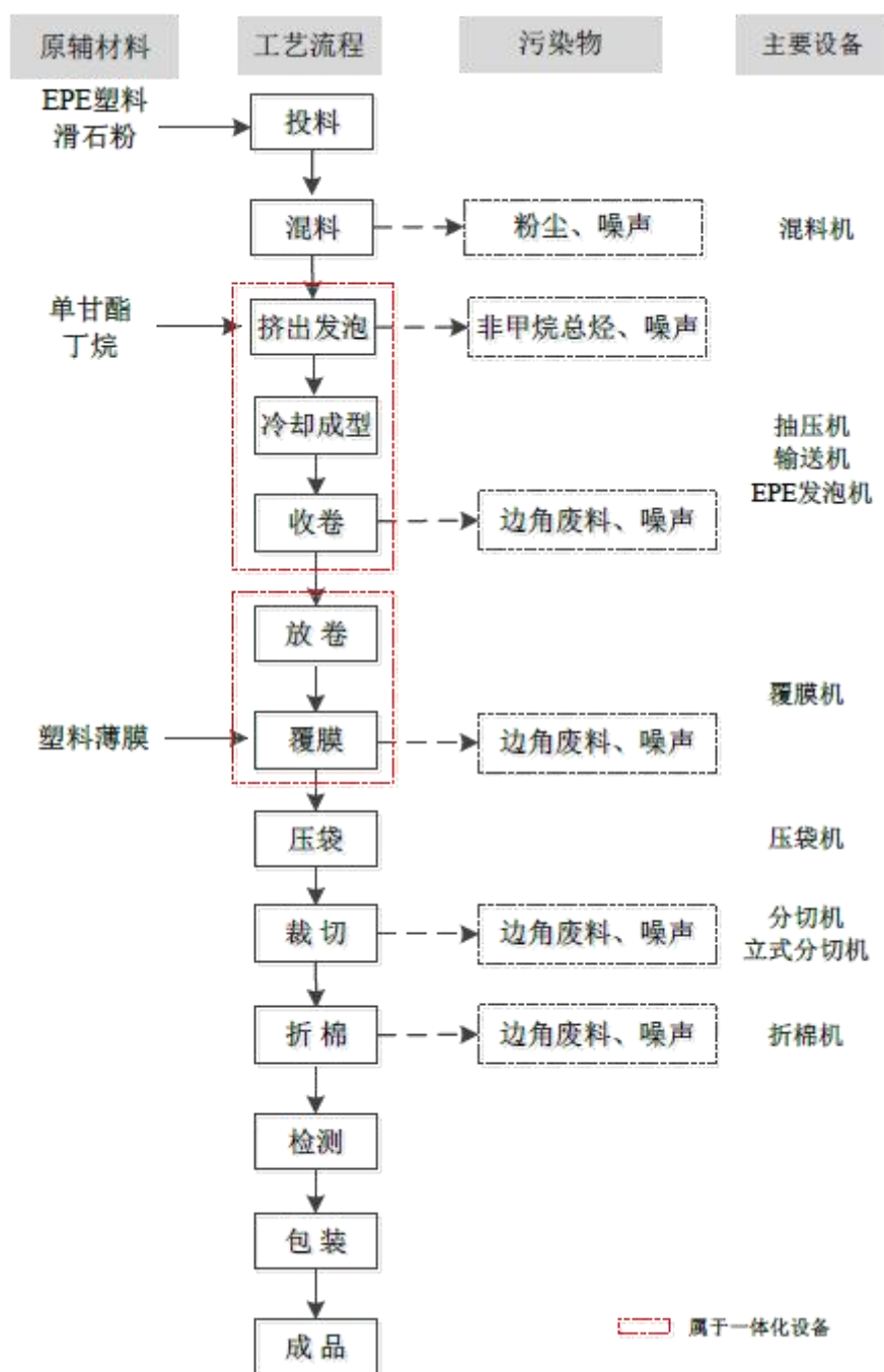
图 3.4-1 生产工艺流程及产污环节图
