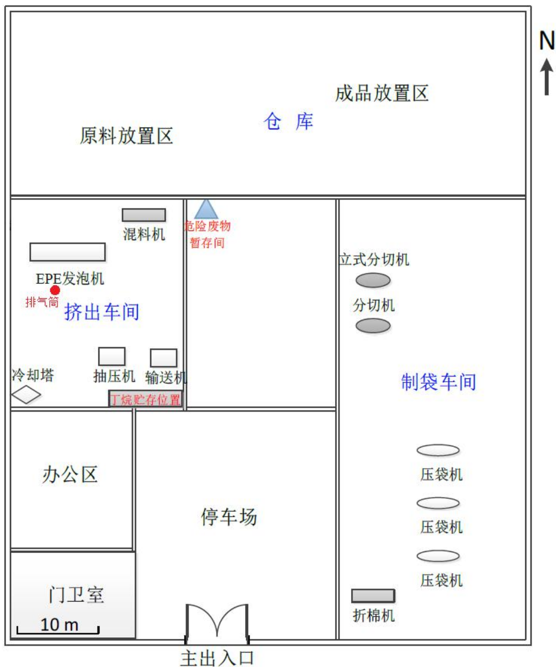
图 3.1-3 平面布置图
