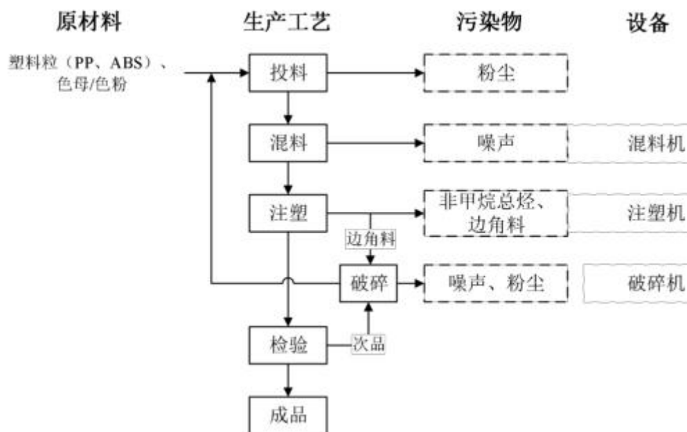
图 3.4-1 生产工艺流程及产污环节图
